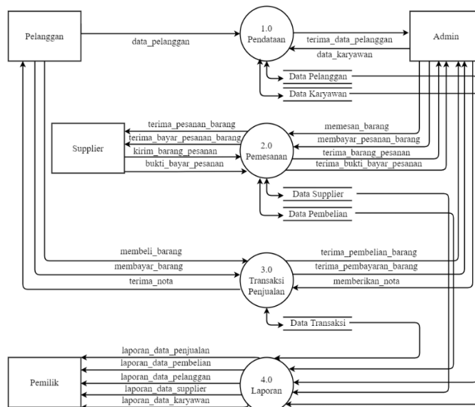
Gambar 2. Diagram Nol Sistem Diusulkan
