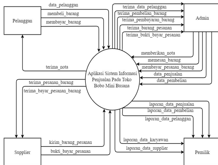
Gambar 1. Diagram Konteks Sistem Diusulkan
